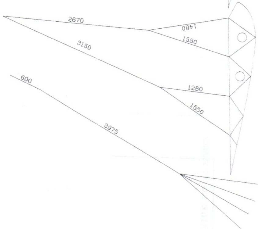
Caisson centraux n° 3 à 7
